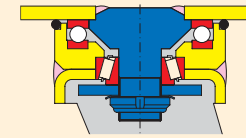
SUPPORTO PESANTE HEAVY DUTY
