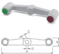
tipi di camma / cam's type
